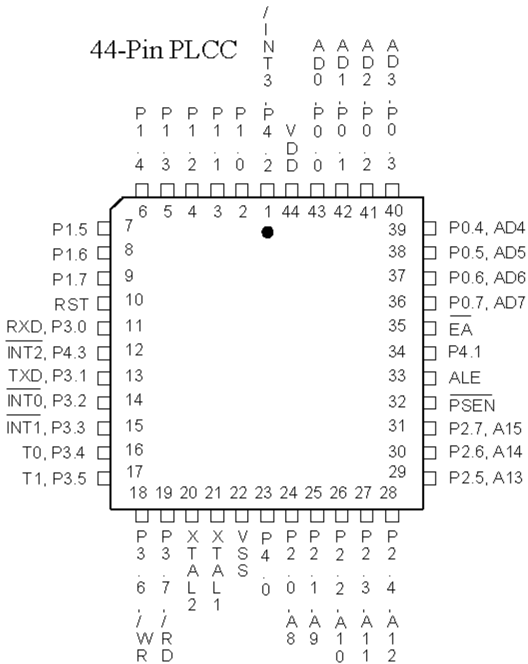
44PIN QFP 封装 51 单片机引脚图
